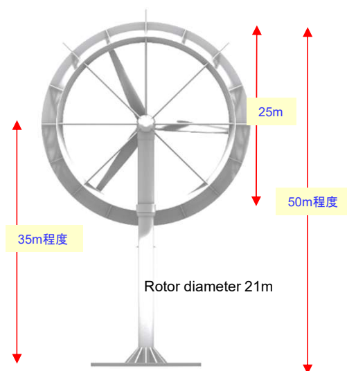
200kWレンズ風車
