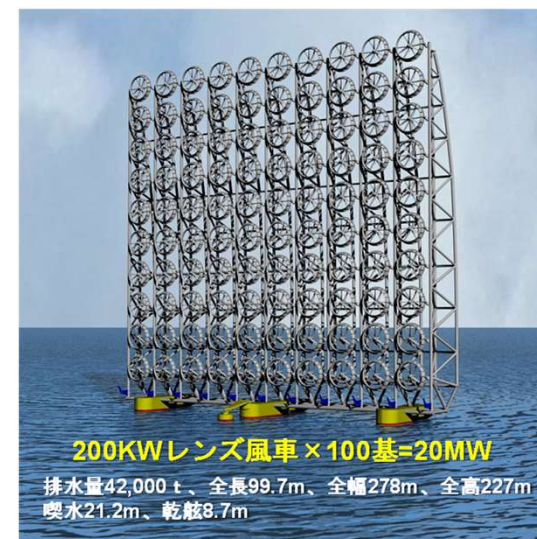
九大RECOW: 将来の20MW マルチレンズ
